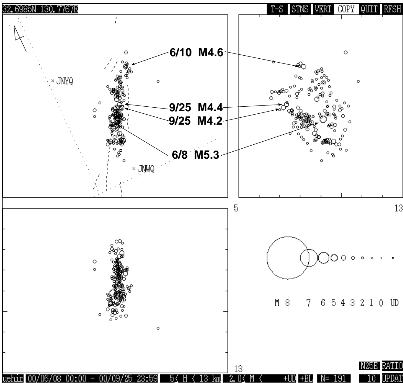
図2 精度の良い震源分布図と発震機構
