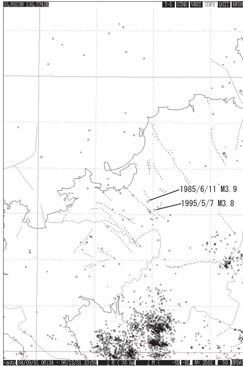
1984年から1996年までの深さ30km以浅の震央分布図
