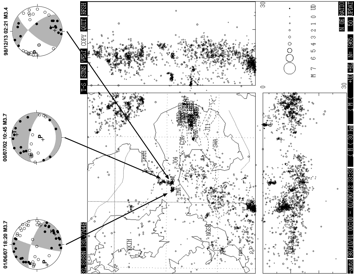
震源分布図(1998/10/1 -2001/6/12)
