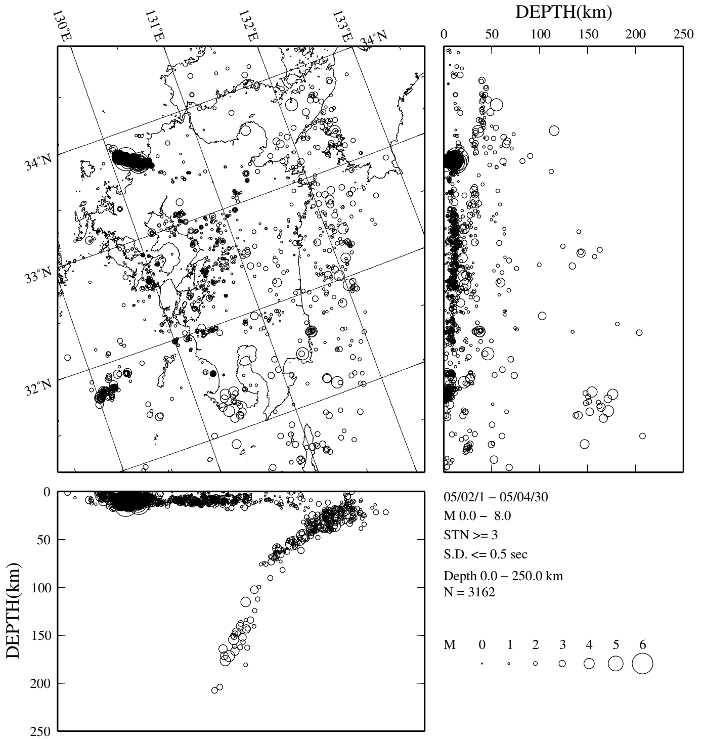
震源分布 (2005年2月~2005年4月)
