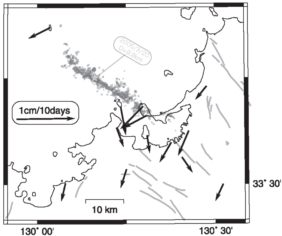
図3. 変動ベクトル図. 座標変化に直線回帰を行い, 10日間の変動率を計算した.
