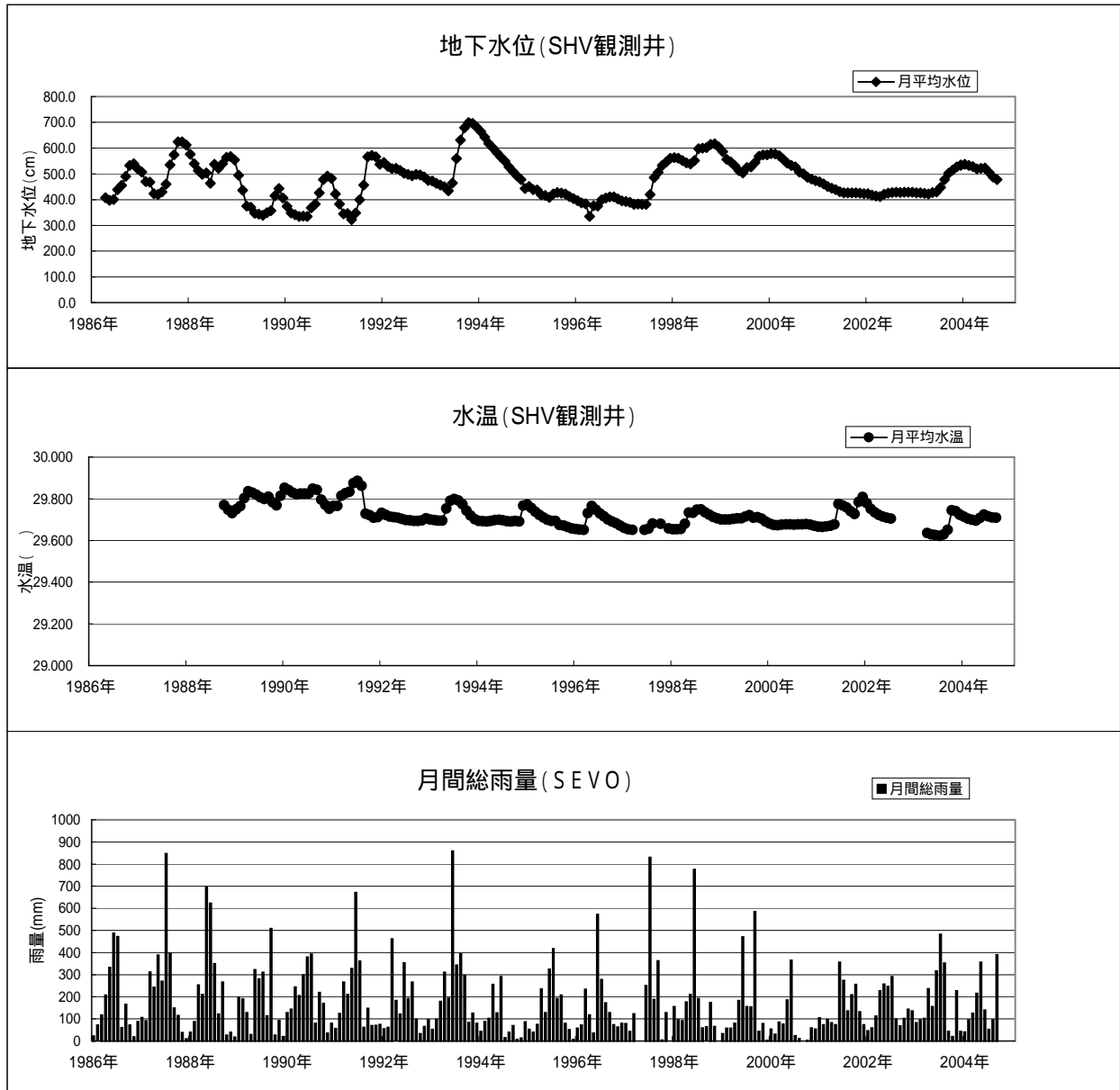
地震火山観測研究センター・島原観測所温泉観測井(SHV観測井)における月平均水位・月平均水温・月間総雨量の観測結果
