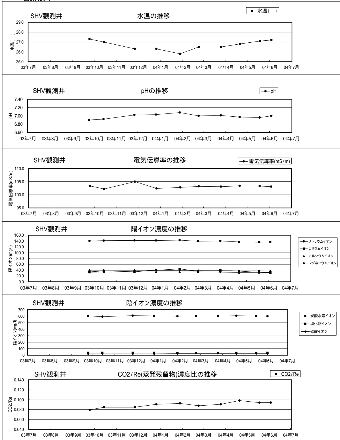
地震火山観測研究センター・島原観測所温泉観測井 (SHV観測井) の温度・pH・電気伝導率・主要化学成分濃度・CO 2 /Re(蒸発残留物)濃度比の推移
