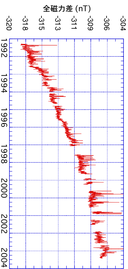
全磁力差 (純差)
