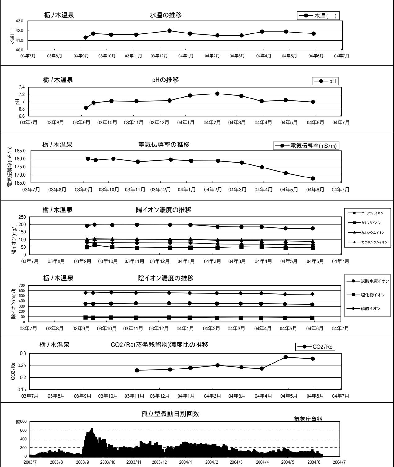
阿蘇栃ノ木温泉小山旅館(平湯)の温度・pH・電気伝導率・主要化学成分濃度・CO 2 /Re(蒸発残留物)濃度比の推移(孤立型微動日別回数は気象庁資料)
