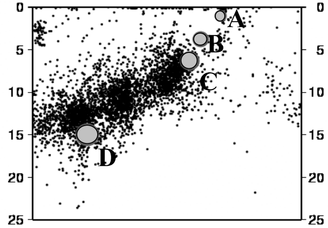
雲仙噴火活動前後の地震活動と 地殻変動圧力源の分布
