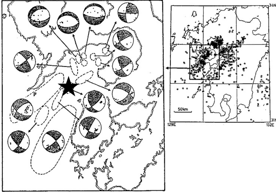
橘湾～天草灘地域の発震機構
