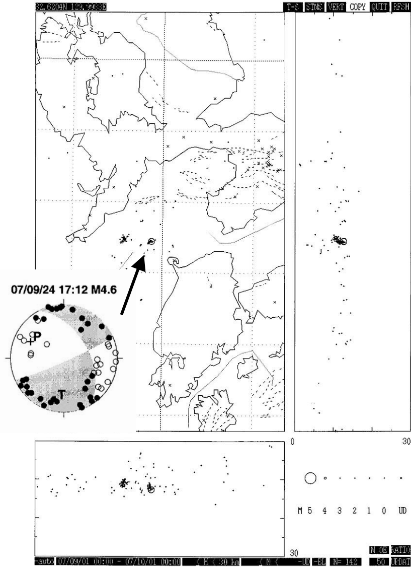
震源分布と最大地震の発震機構
