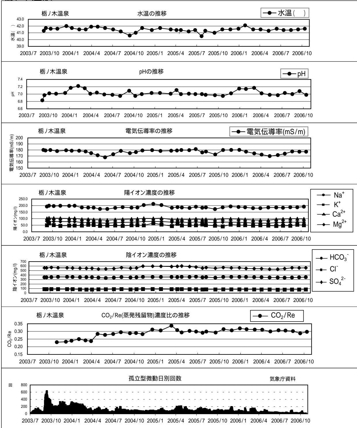
阿蘇栃ノ木温泉小山旅館(平湯)の水温・pH・電気伝導率・主要化学成分濃度・CO 2 /Re(蒸発残留物)濃度比の推移 (孤立型微動日別回数は気象庁資料)
